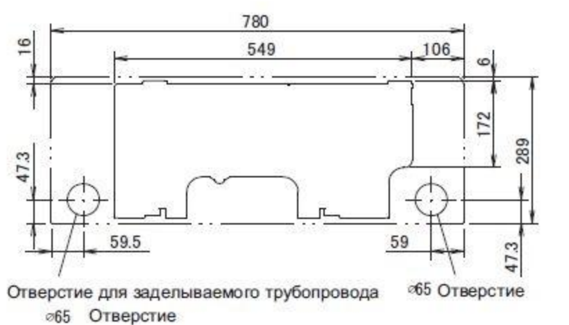
Стандартное расположение отверстий в стене
